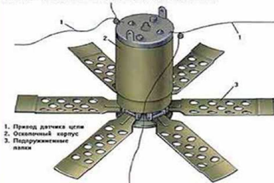
Мина ПОМ-2Р в боевом положении
